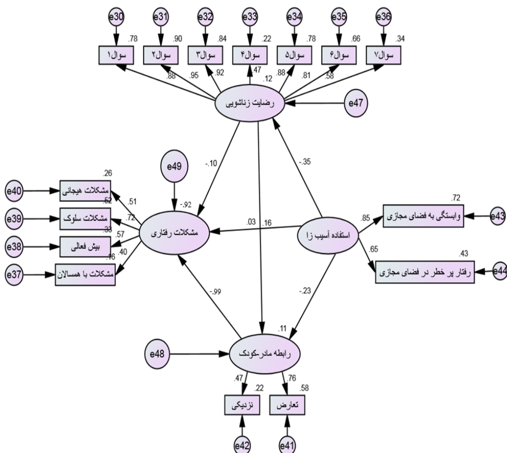
شکل ۱: ضرایب استاندارد مدل پیشنهادی برای بررسی مدل معادلات ساختاری پیشنهادی پژوهش
