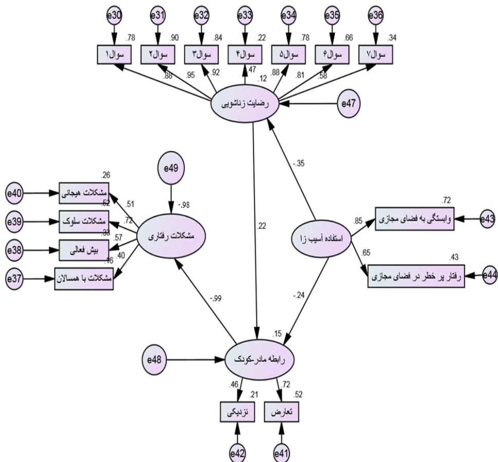
شکل ۲: مدل اصلاح شده بر اساس حذف مسیرهای غیر معنادار
